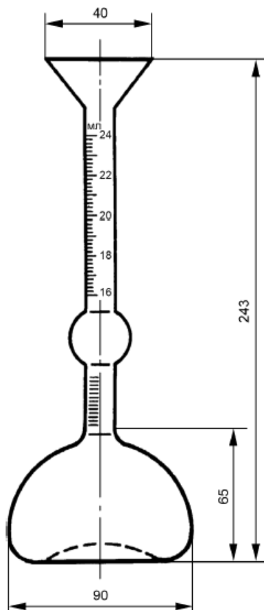
Прибор Ле-Шателье
